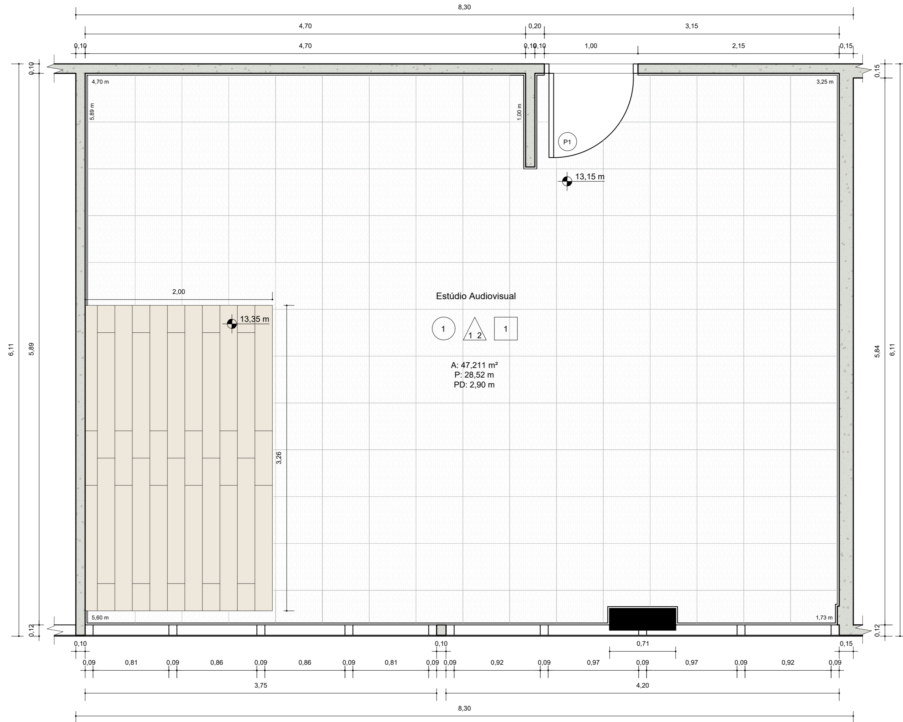
4 PLANTA BAIXA - PISO ESCALA 1:25
